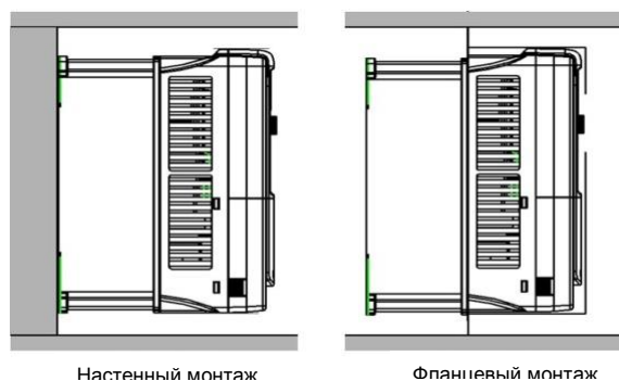
Рис. 4-1 Установка ПЧ
