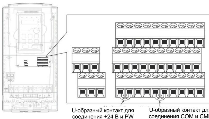
Рис.5-18 U-образный контакт
