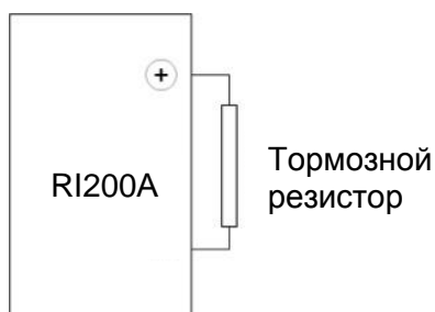
Рис. 12-5. Схема подключения тормозного резистора
