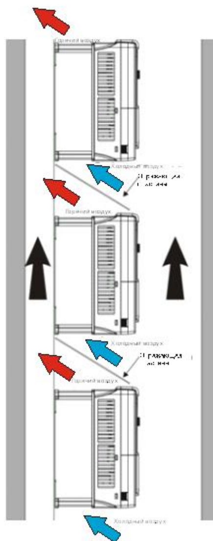
Рис. 4-4 Вертикальная установка
