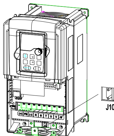
Рис. 12-3. Схема подключения ЭМС-фильтра С3
